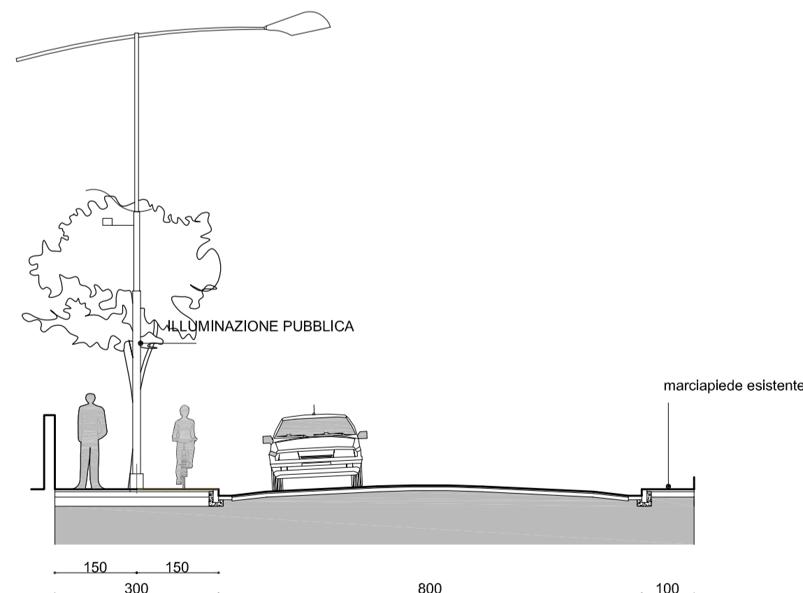
SEZIONE A-A
